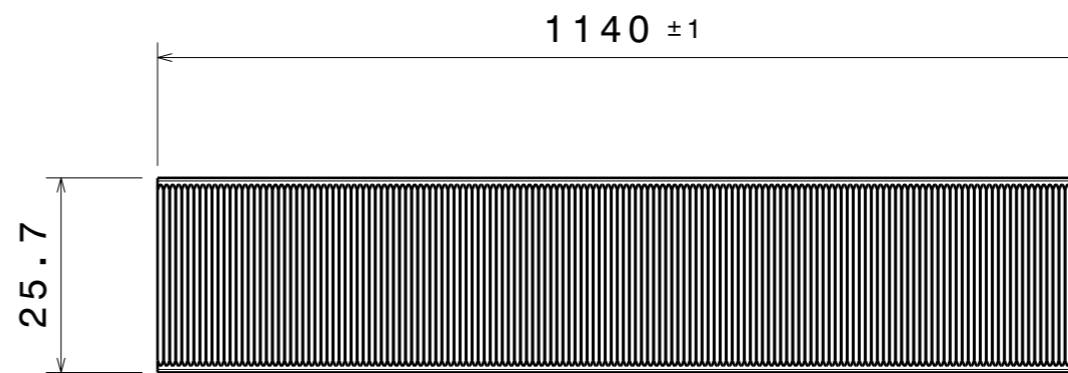
Left view Scale: 1:1
